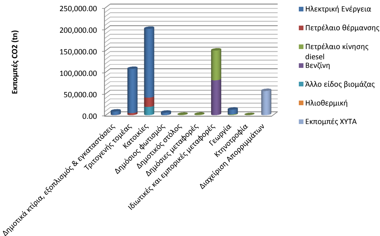
Σχήμα 0.2: Τελικές εκπομπές CO 2 ανά πηγή και ανά τομέα (2013)
