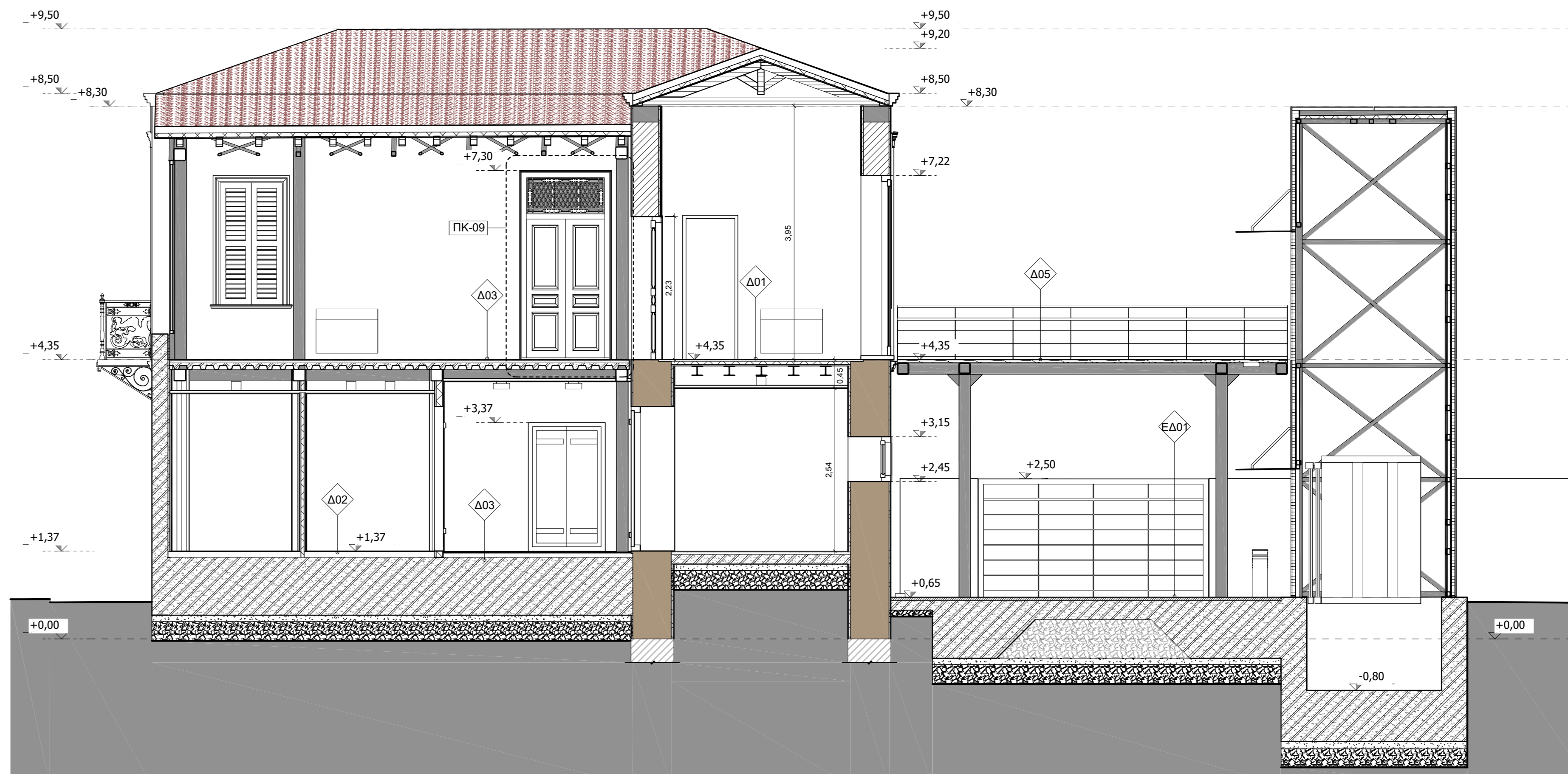
TOMH Δ-Δ
