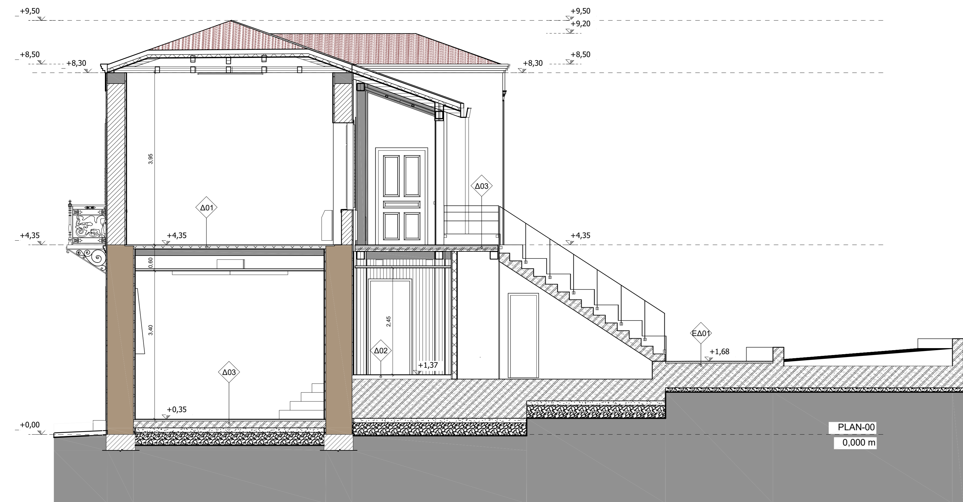
TOMH A-A
