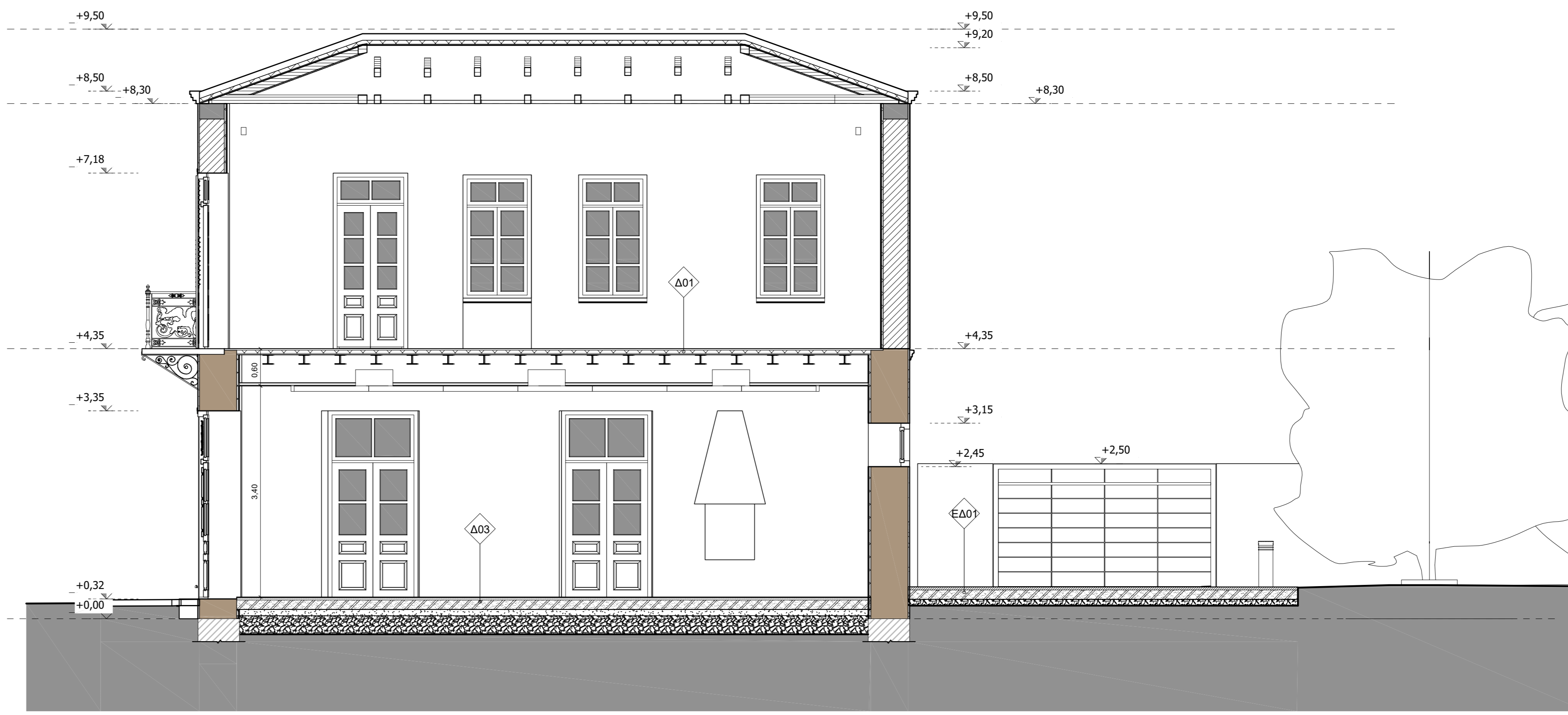
TOMH Γ-Γ
